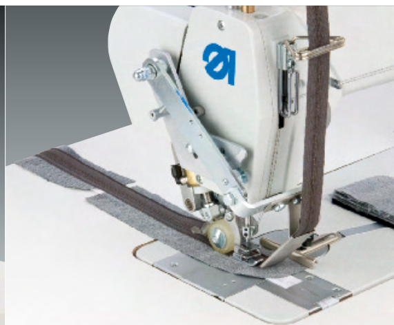
Parts Set 550-2-2, E204/5
